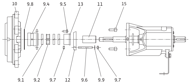
Fig. 21: Исполнение с сальниковым уплотнением
